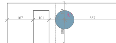
POGLED NA ZID 2-2
