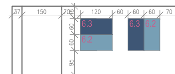
POGLED NA ZID 6-6
